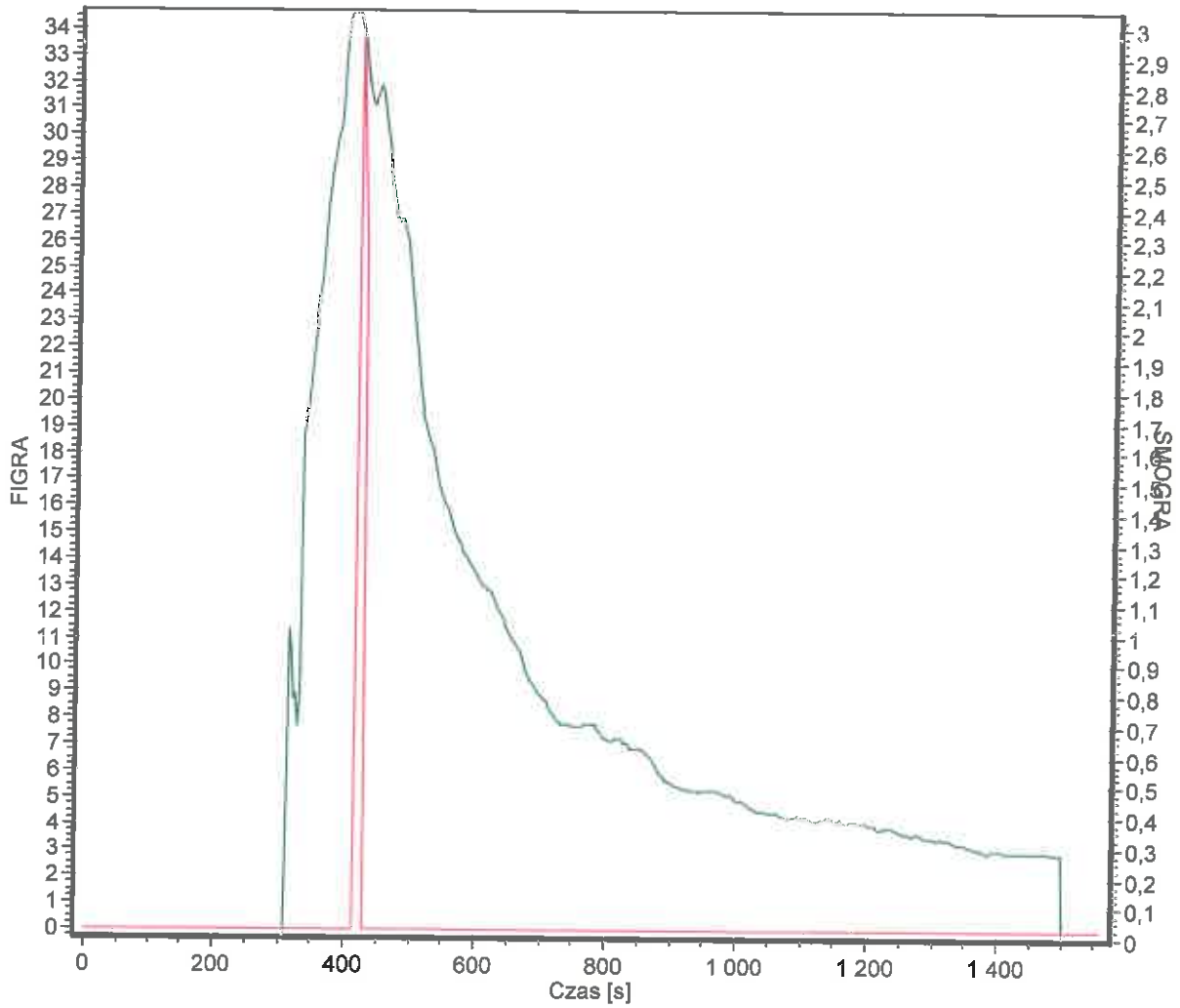
Wykres HRRav(t)/(t-300) oraz SPRav(t)/(t-300)
