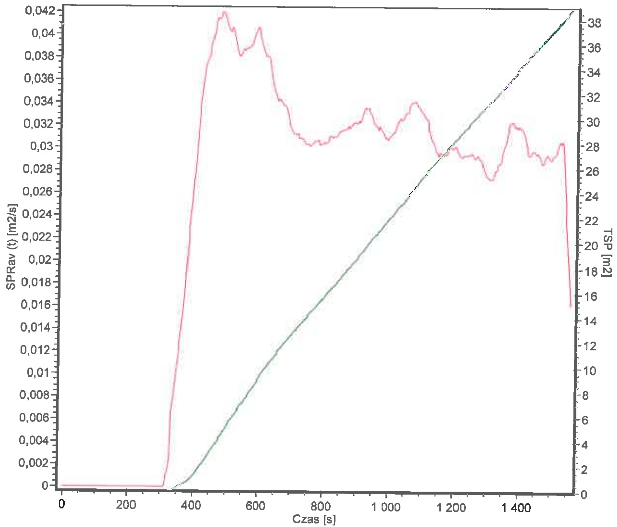
Wykres SPR oraz TSP
