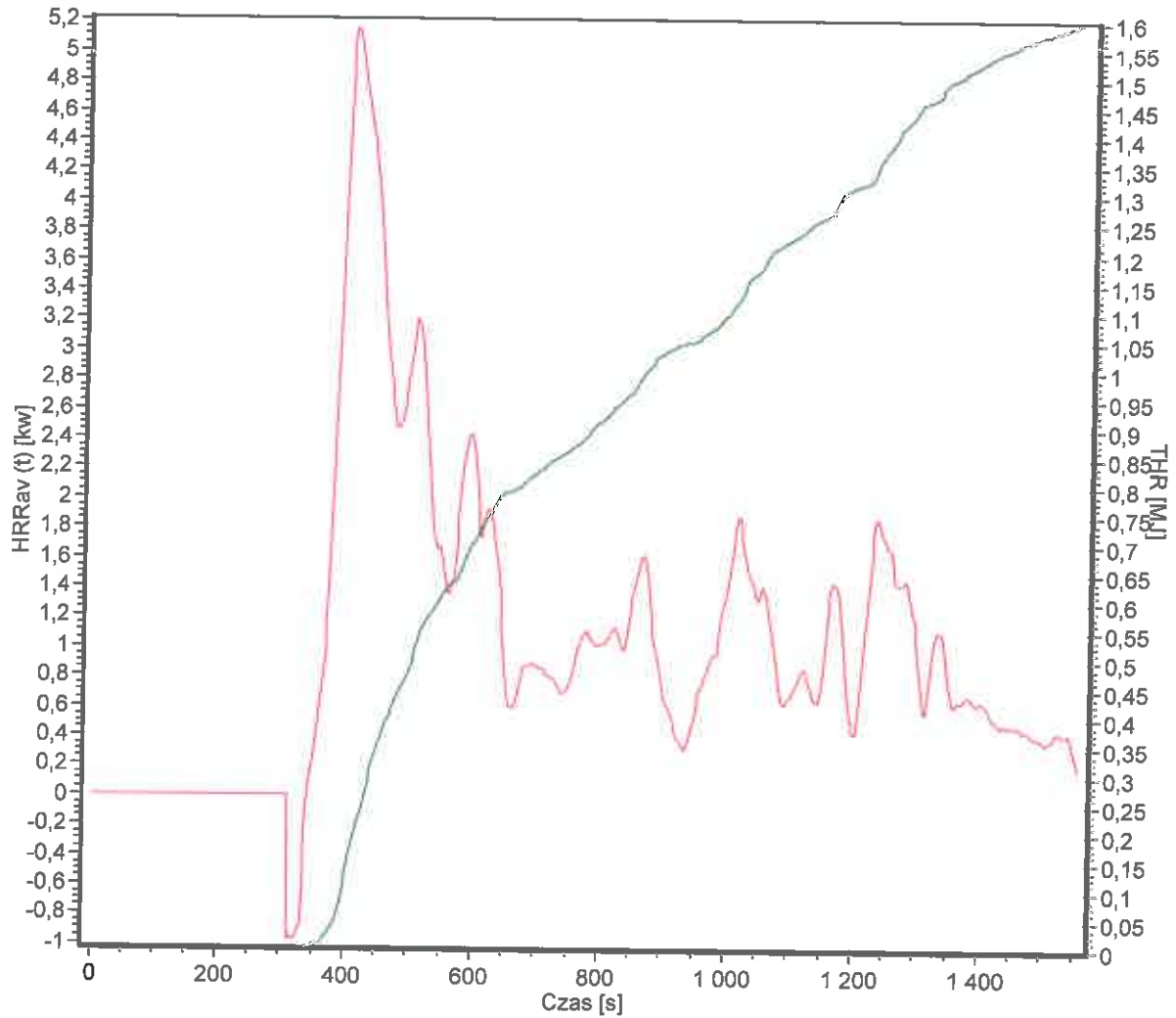
Wykres HRR oraz THR
